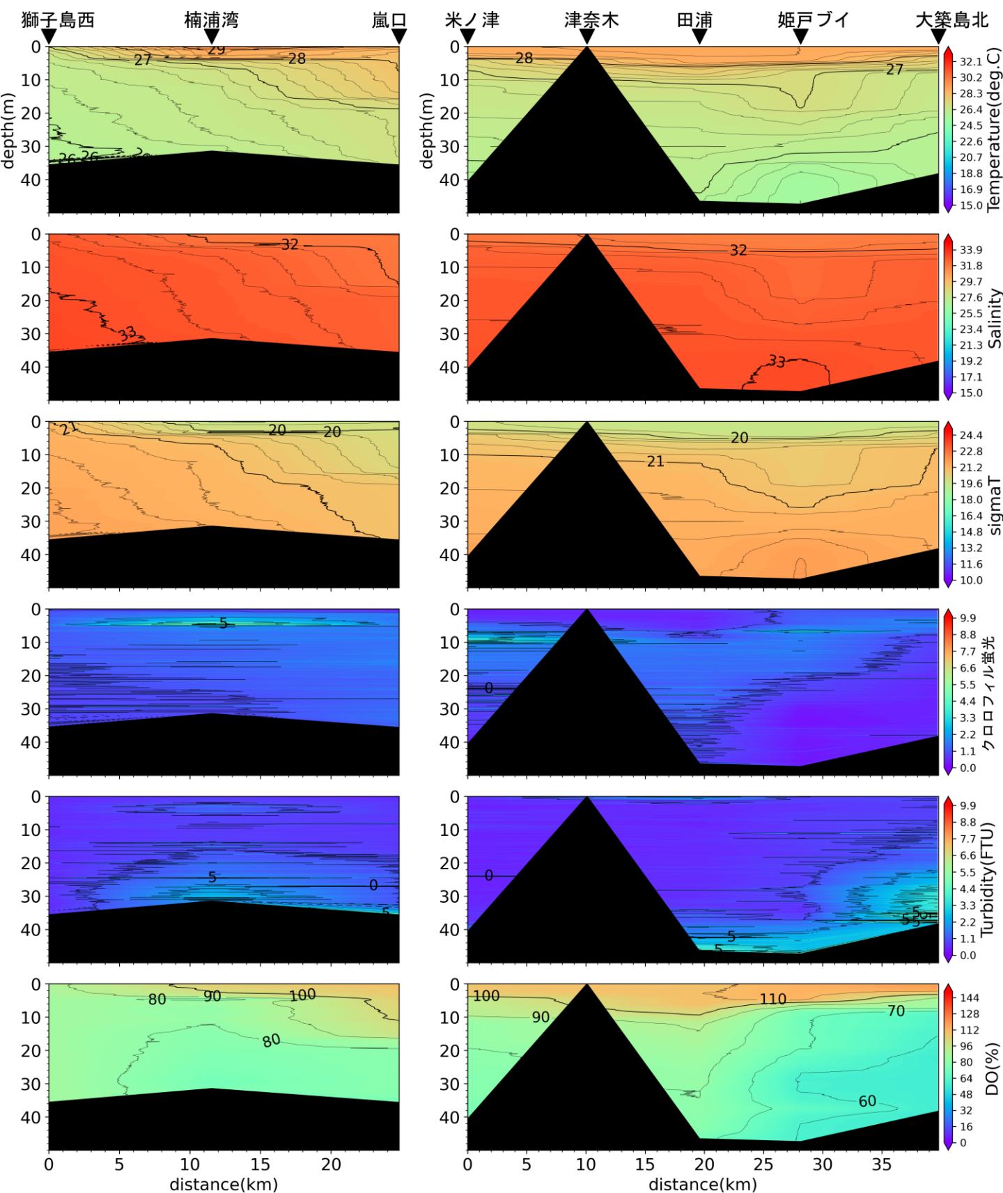
嵐口から獅子島西, 大築島北から米ノ津の水温(°C)、塩分、密度( \sigma_t )、クロロフィル蛍光強度、濁度、溶存酸素飽和度(DO%)の鉛直面図(東町漁業協同組合の調査による)(2025年9月9日)
