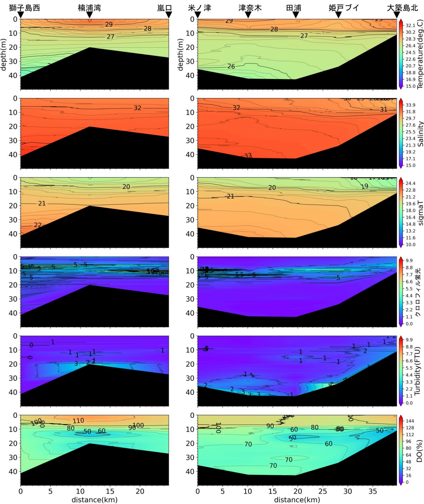
嵐口から獅子島西, 大築島北から米ノ津の水温(°C)、塩分、密度( \sigma_t )、クロロフィル蛍光強度、濁度、溶存酸素飽和度(DO%)の鉛直面図(熊本県水産研究センターの調査による)(2025年9月2日)
