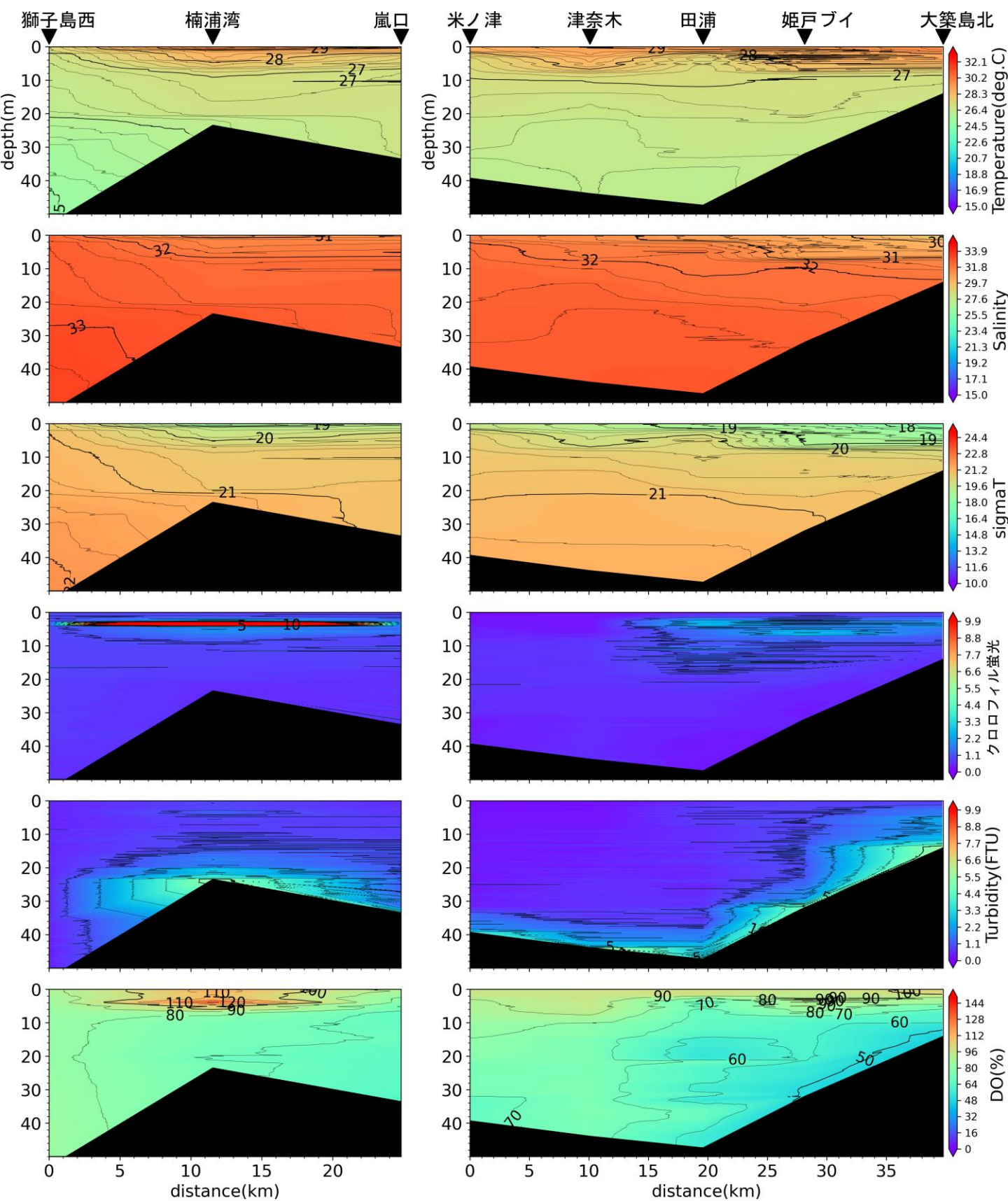
嵐口から獅子島西, 大築島北から米ノ津の水温(°C)、塩分、密度( \sigma_t )、クロロフィル蛍光強度、濁度、溶存酸素飽和度(DO%)の鉛直面図(鹿児島県水産技術開発センターの調査による)(2025年8月26日)
