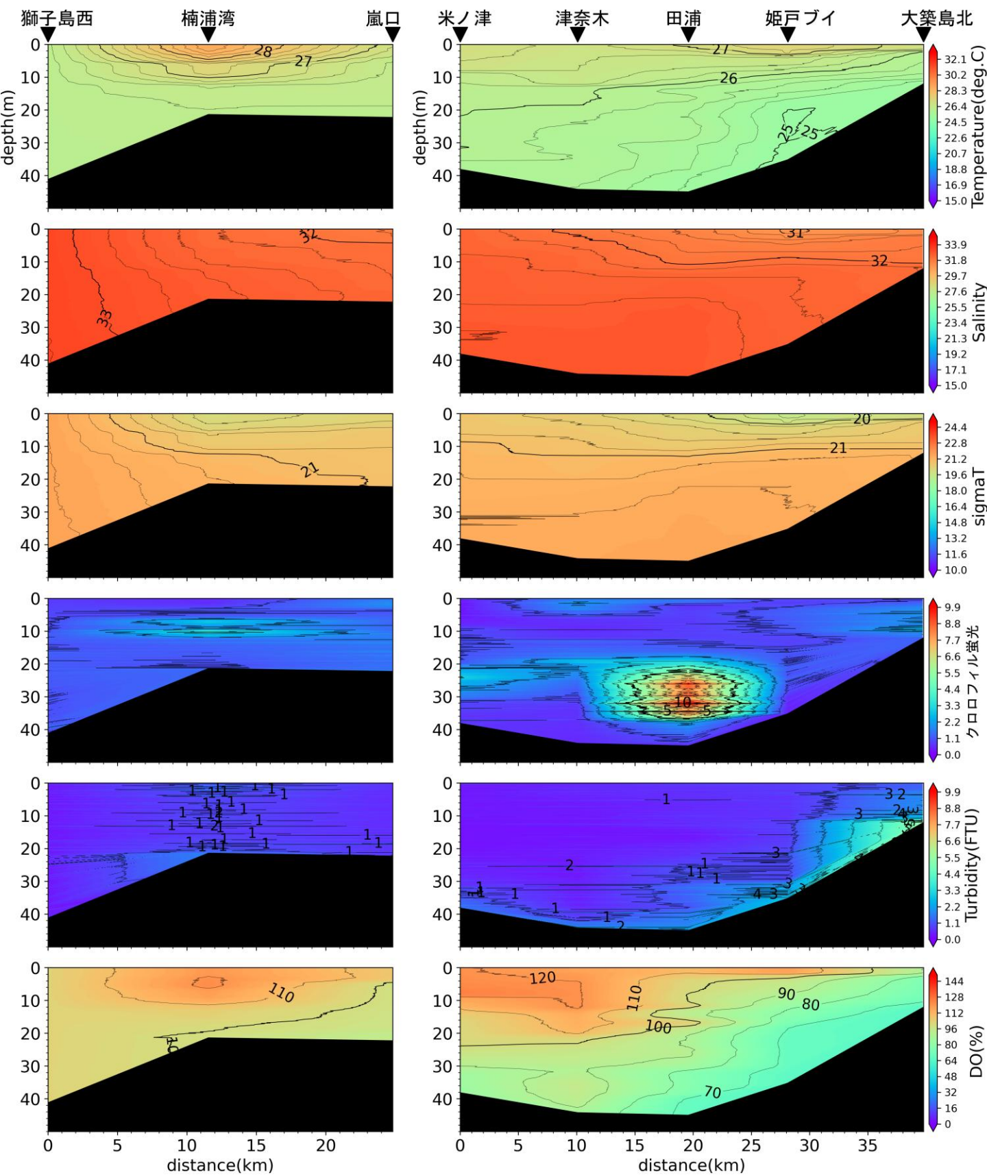
嵐口から獅子島西, 大築島北から米ノ津の水温(°C)、塩分、密度( \sigma_t )、クロロフィル蛍光強度、濁度、溶存酸素飽和度(DO%)の鉛直面図(熊本県水産研究センターの調査による)(2025年7月29日)
