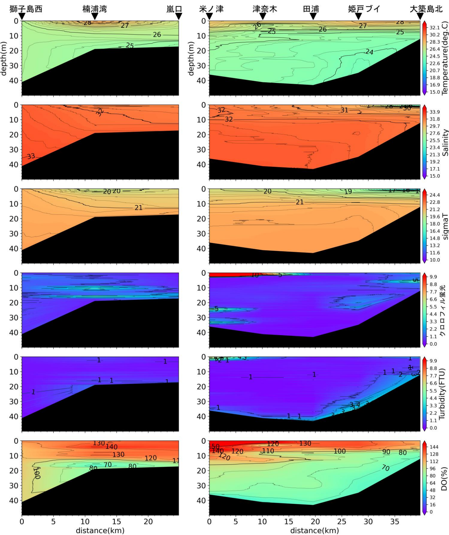
嵐口から獅子島西, 大築島北から米ノ津の水温(°C)、塩分、密度( \sigma_t )、クロロフィル蛍光強度、濁度、溶存酸素飽和度(DO%)の鉛直面図(熊本県水産研究センターの調査による)(2025年7月22日)
