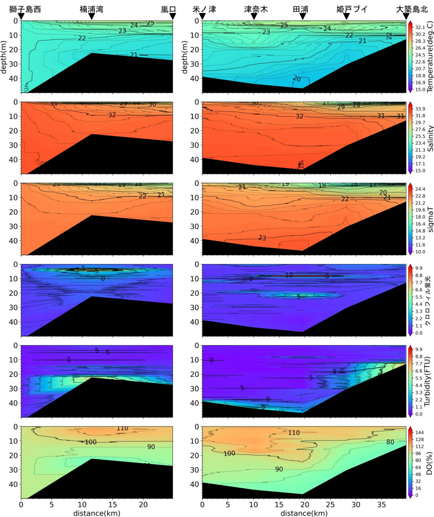
嵐口から獅子島西, 大築島北から米ノ津の水温(°C)、塩分、密度( \sigma_t )、クロロフィル蛍光強度、濁度、溶存酸素飽和度(DO%)の鉛直面図(鹿児島県水産技術開発センターの調査による)(2025年6月24日)
