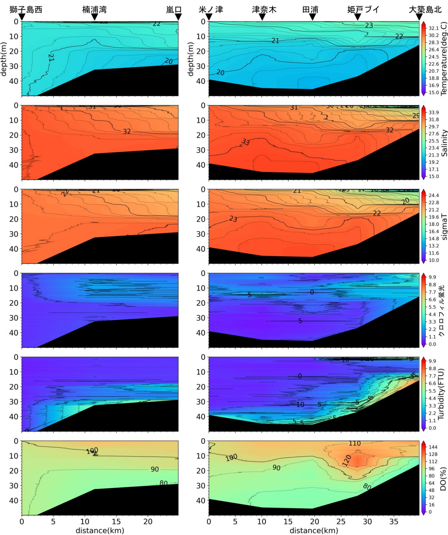
嵐口から獅子島西, 大築島北から米ノ津の水温(°C)、塩分、密度( \sigma_t )、クロロフィル蛍光強度、濁度、溶存酸素飽和度(DO%)の鉛直面図(東町漁業協同組合の調査による)(2025年6月17日)
