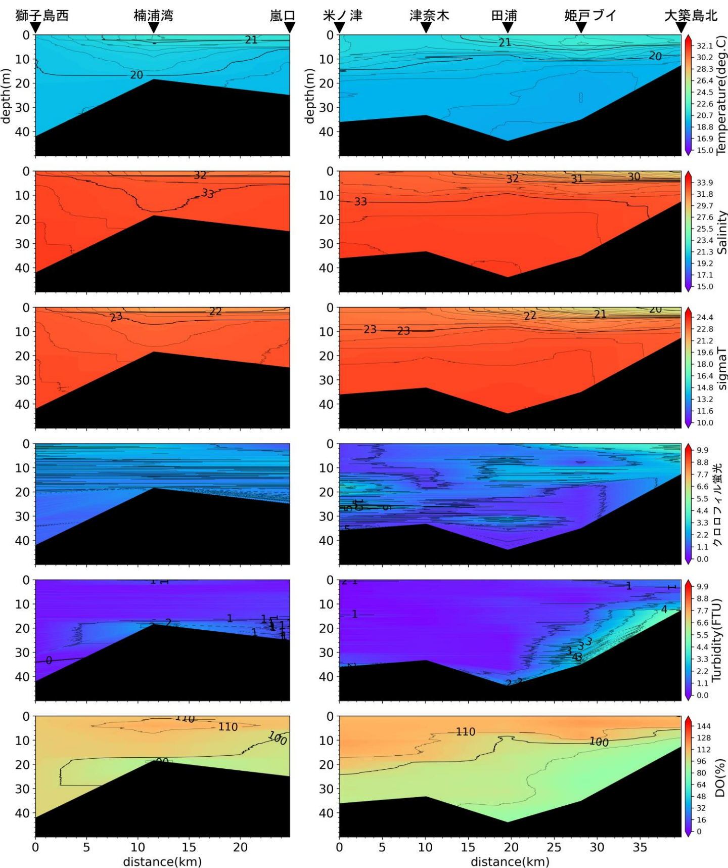
嵐口から獅子島西, 大築島北から米ノ津の水温(°C)、塩分、密度( \sigma_t )、クロロフィル蛍光強度、濁度、溶存酸素飽和度(DO%)の鉛直面図(熊本県水産研究センターの調査による)(2025年6月9日)
