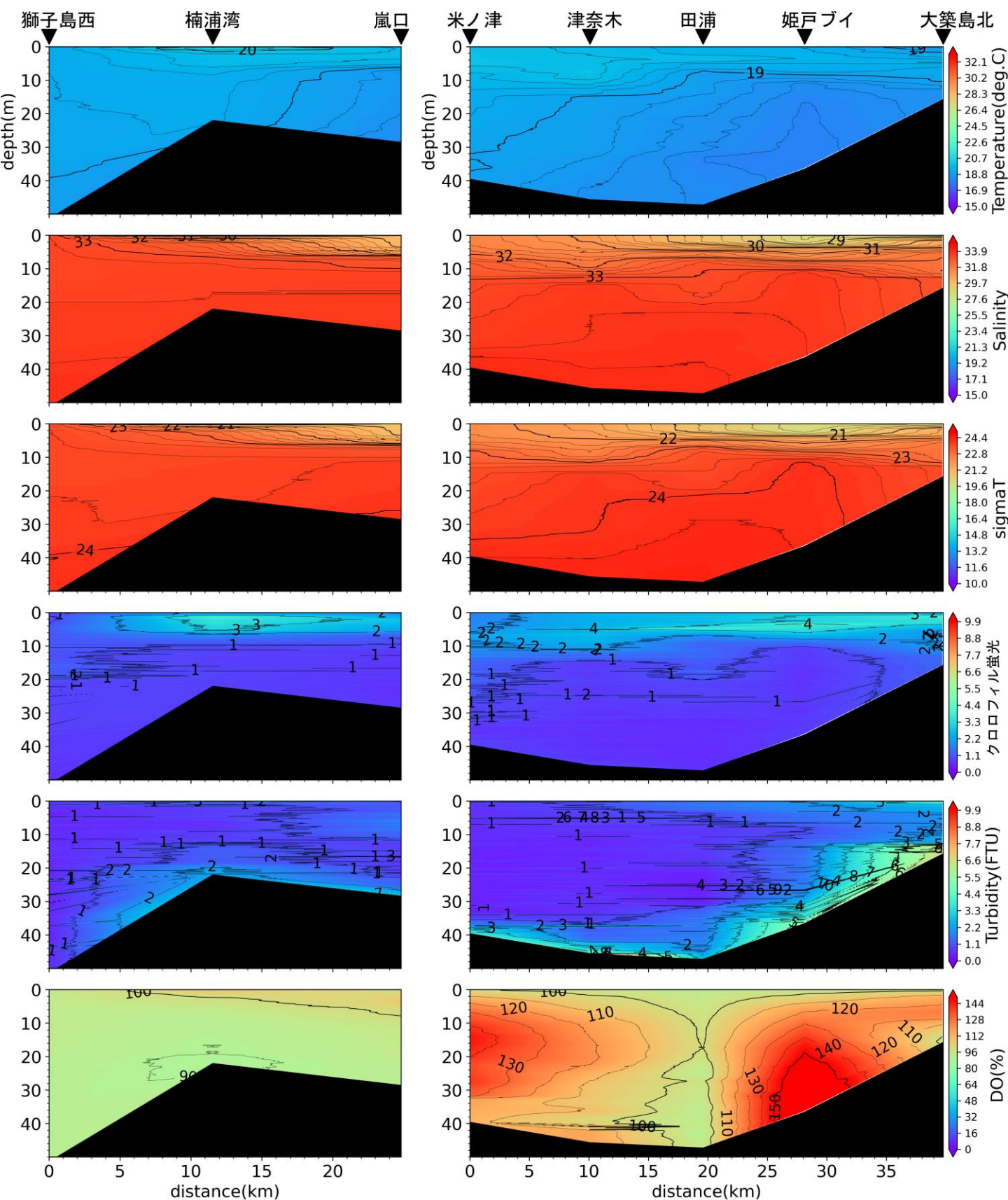
嵐口から獅子島西，大築島北から米ノ津の水温(°C)、塩分、密度( \sigma_t )、クロロフィル蛍光強度、濁度、溶存酸素飽和度(DO%)の鉛直面図(東町漁業協同組合の調査による)(2025年5月26日)
