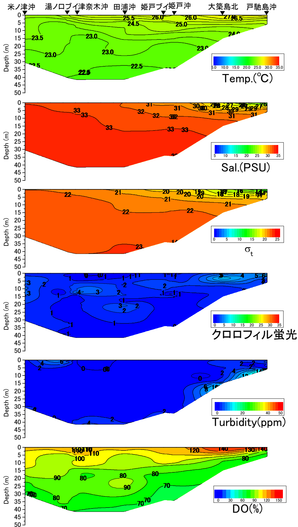
戸馳島沖から米ノ津沖の水温(°C)、塩分、密度( \sigma_t )、クロロフィル蛍光強度、濁度、溶存酸素飽和度(DO%)の鉛直面図(東町漁業協同組合の調査による) (2013年7月8日)
