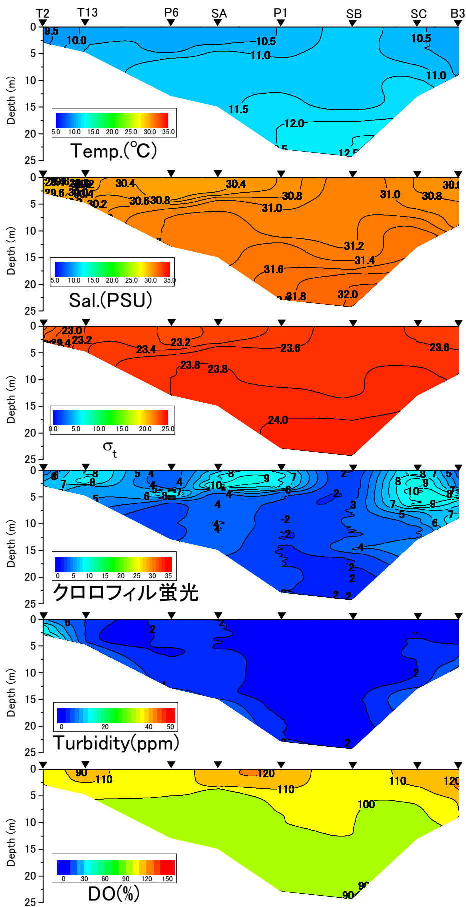
2019年1月15日にける水温、塩分、密度 \sigma_t 、クロロフィル蛍光値、濁度、DO飽和度
