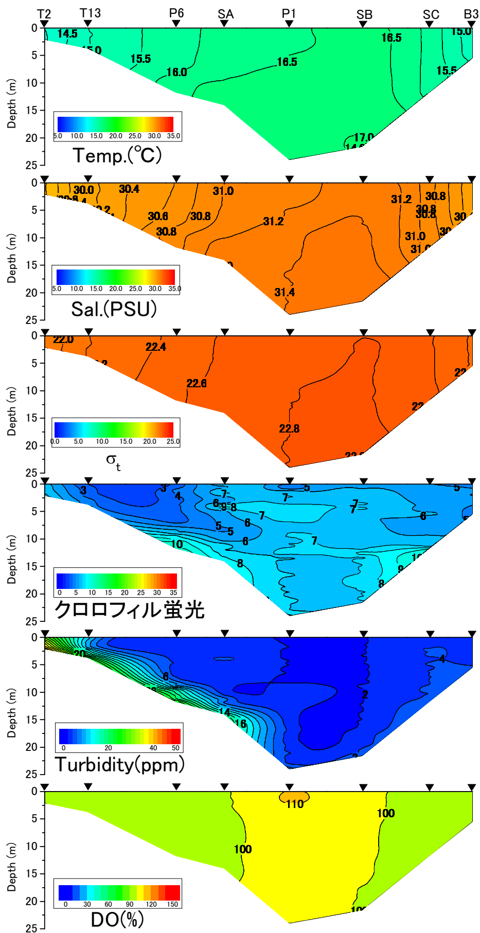
2018年11月29日にける水温、塩分、密度 \sigma_t 、クロロフィル蛍光値、濁度、DO飽和度
