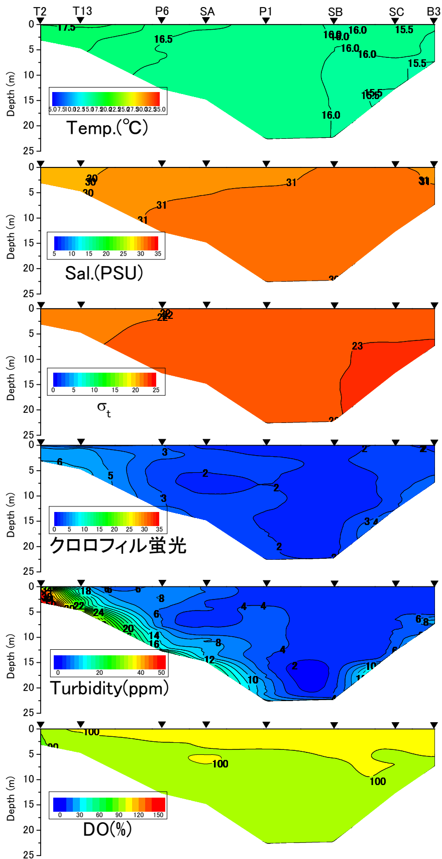
2013年5月1日における水温、塩分、密度 \sigma_t 、クロロフィル蛍光値、濁度、DO飽和度
