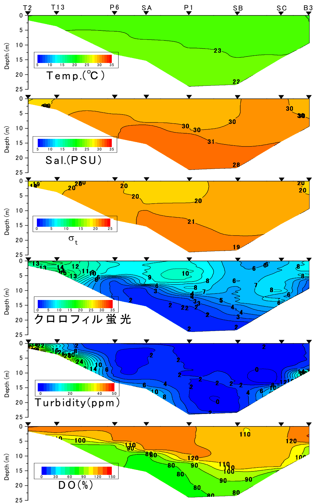
有明海湾奥西部海域の水質の断面分布（2012年10月11日）
