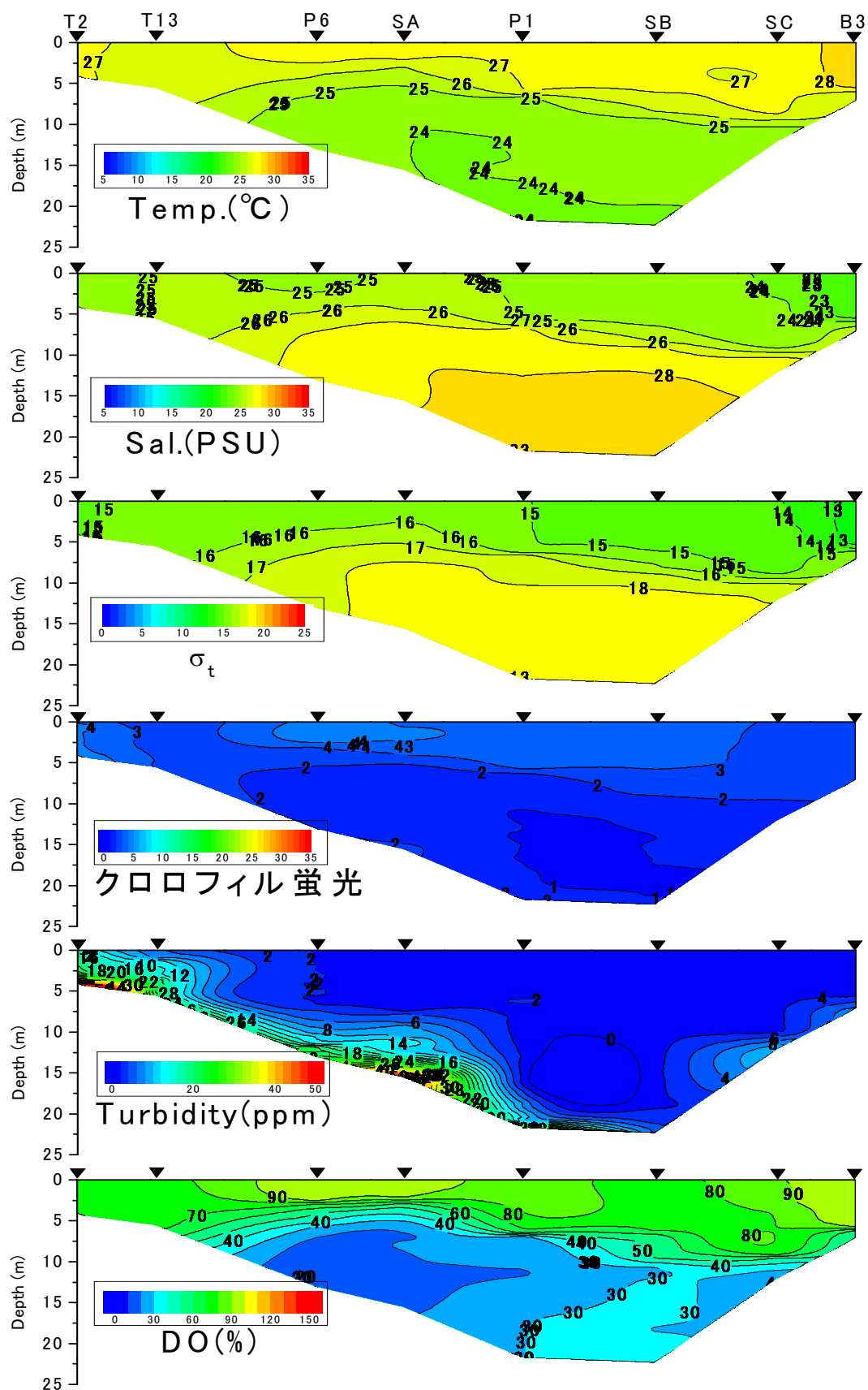
有明海湾奥西部海域の水質の断面分布（2012年8月5日）
