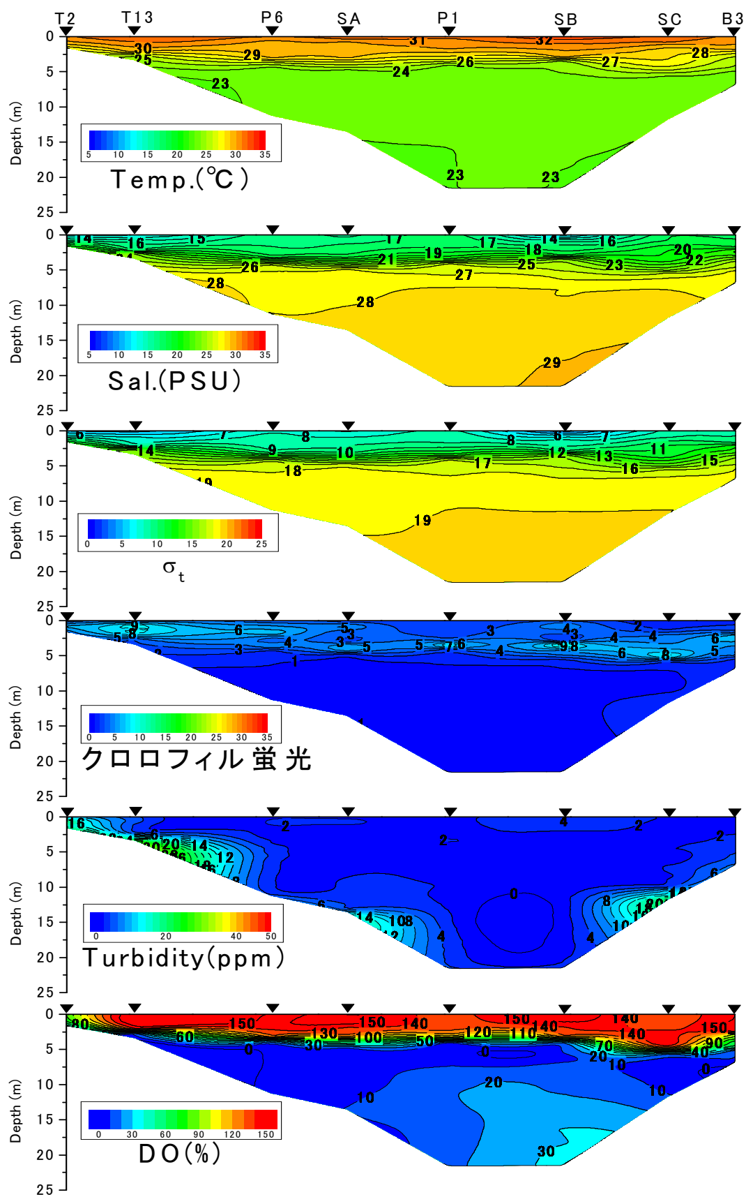
有明海湾奥西部海域の水質の断面分布（2012年7月29日）
