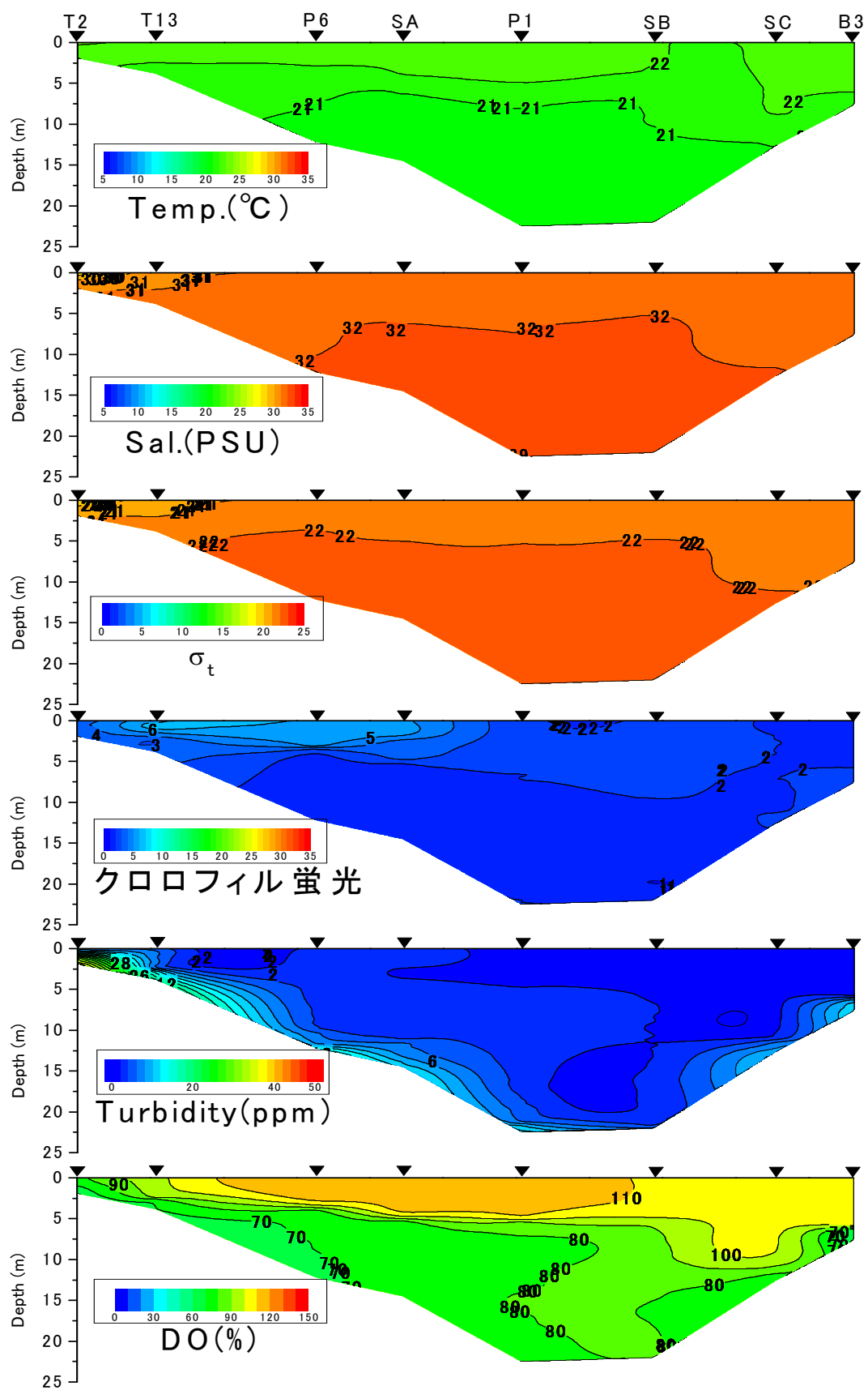
有明海湾奥西部海域の水質の断面分布（2012年6月12日）
