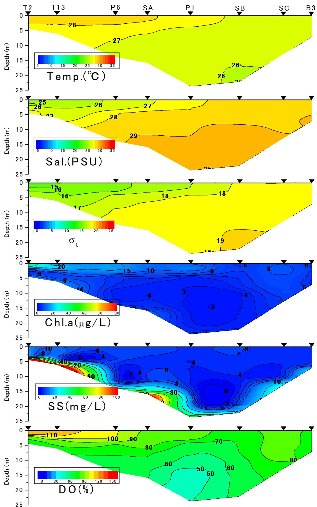
有明海湾奥西部海域の水質の断面分布（2011年8月17日）
