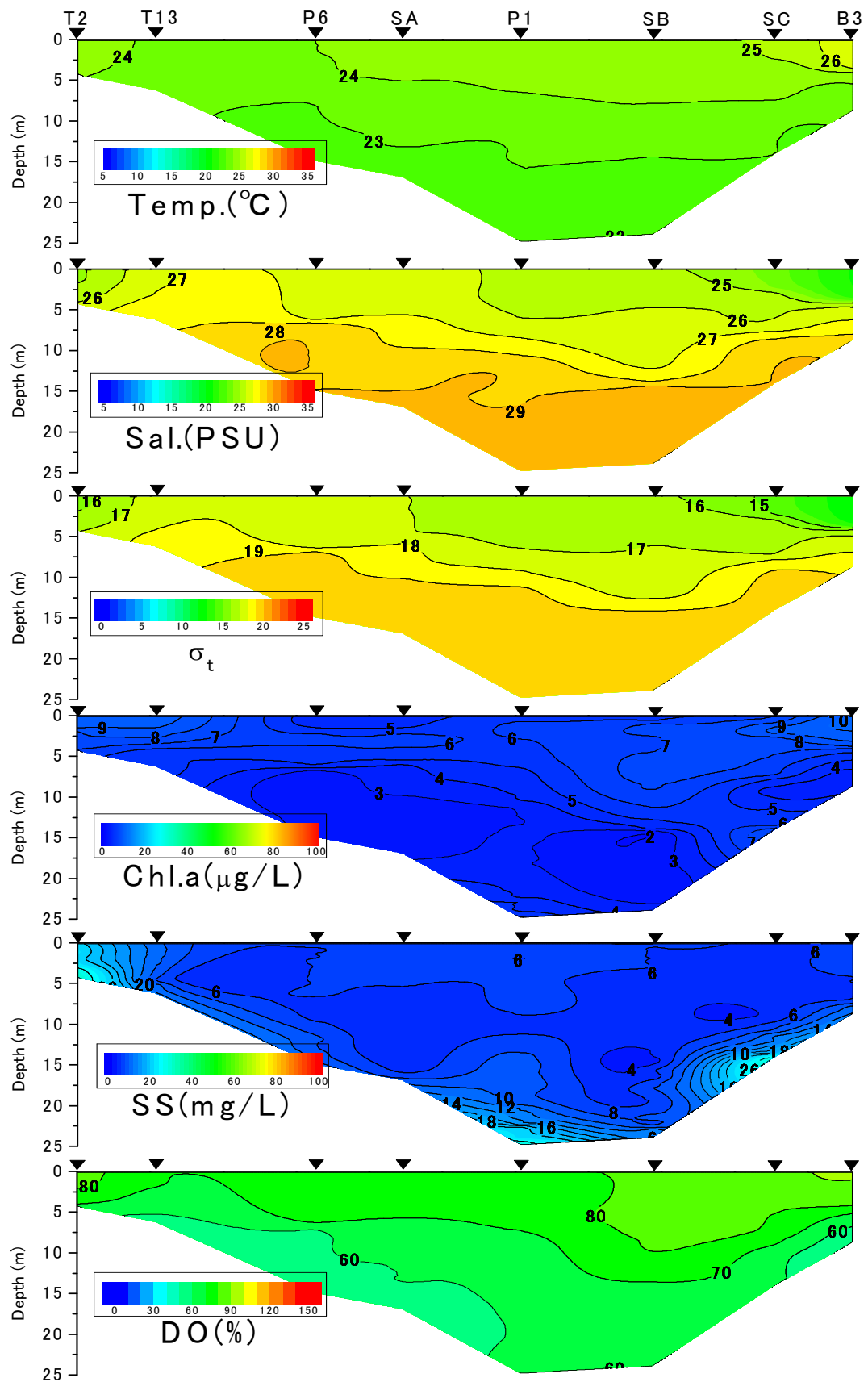
有明海湾奥西部海域の水質の断面分布（2011年7月20日）
