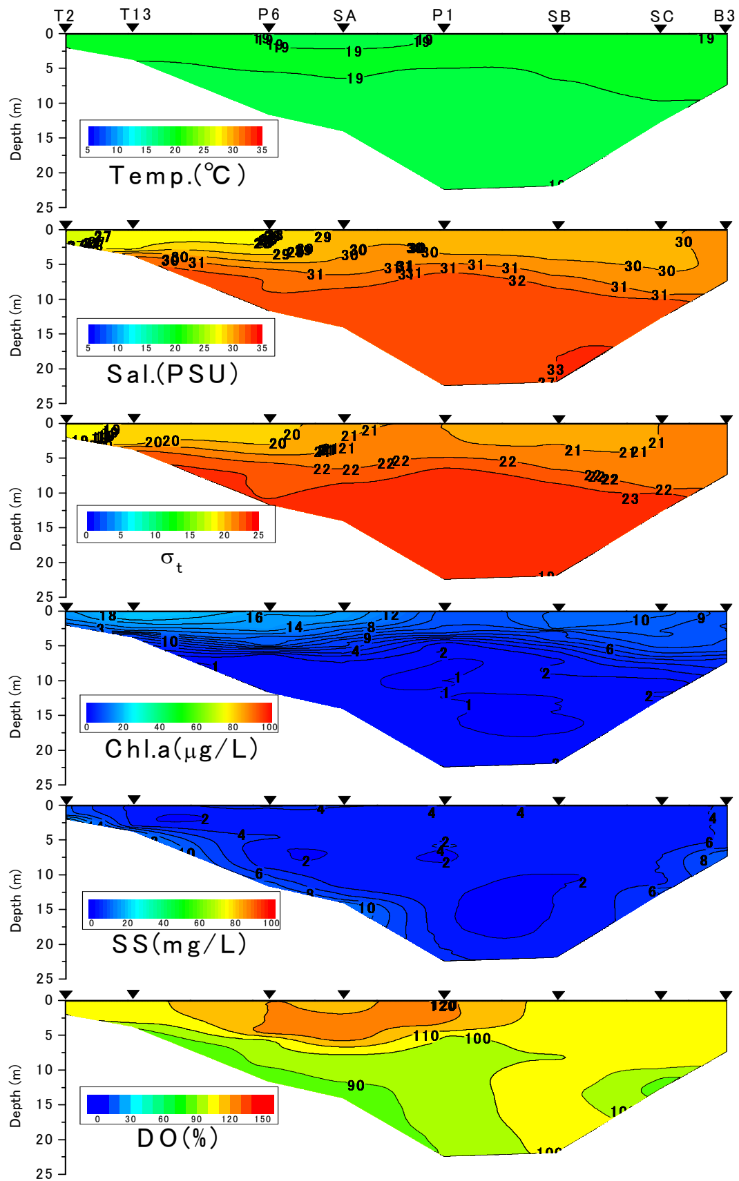
有明海湾奥西部海域の水質の断面分布（2011年5月26日）
